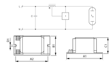
Technische Daten Philips BSN 250 semi-paralleles Vorschaltgerät L33-A4 | SON-CDO-MH-HPI - 230V Produkt ansehen
